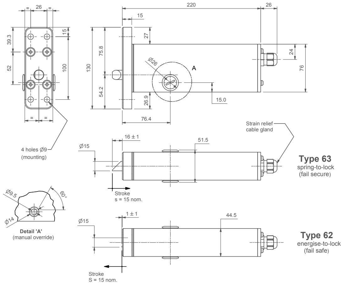
Fig. 4 Dimensions
